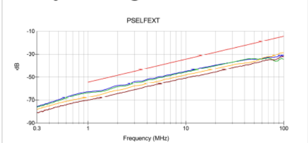
Limit Margin : 8.500 dB @ 1.001 MHz
